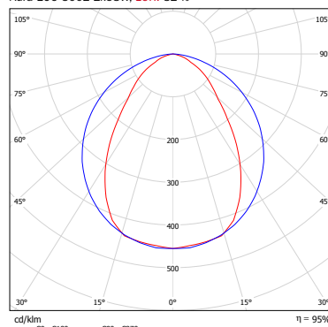
Aura ECO 3002 2x58W, LOR: 82 %
