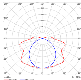
Aura ECO 2003 2x28W, LOR: 86 %
