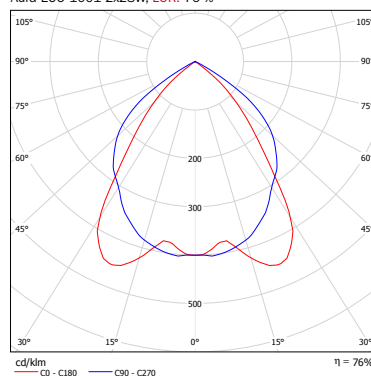
Aura ECO 1001 2x28W, LOR: 76 %
