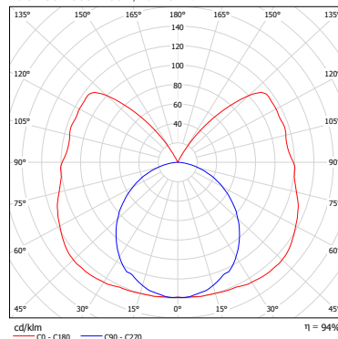
Aura ECO 1003 1x35W, LOR: 94 %
