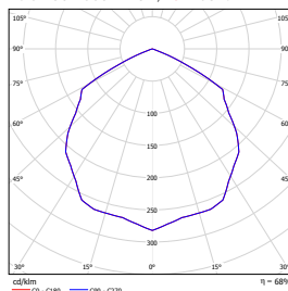
Aura ECO 1503 2x18W, LOR: 61 %
