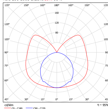
Aura ECO 1003 1x28W, LOR: 95 %
