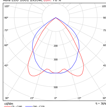
Aura ECO 1001 2x35W, LOR: 76 %
